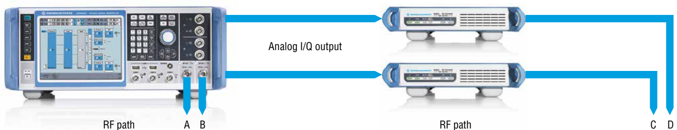
Измерительная установка для 4x4 МИМО, состоящая из двухканального генератора R&S®SMW200A и двух модулей генерации сигналов R&S®SGS100A, управляемых с генератора R&S®SMW200A. Модули обеспечивают ВЧ-тракты 3 и 4. Генератор R&S®SMW200A полностью обеспечивает систему модулирующим сигналом и замираниями
